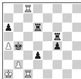
452 L. Kubbel, 1928
