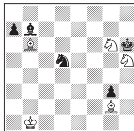
456 A. Malisjev, 1987
